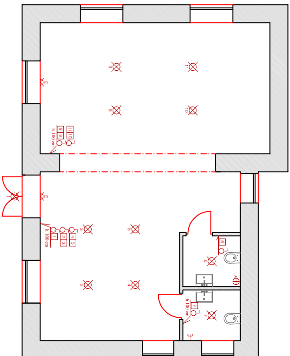
PIANTA PIANO TERRA Scala 1:50
